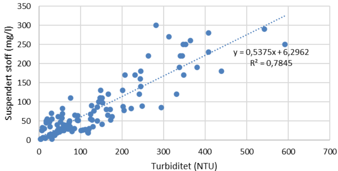
Suspendert stoff vs turbiditet
