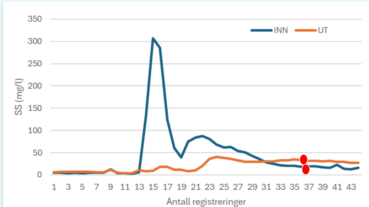
Omregnet til suspendert stoff inn og ut
