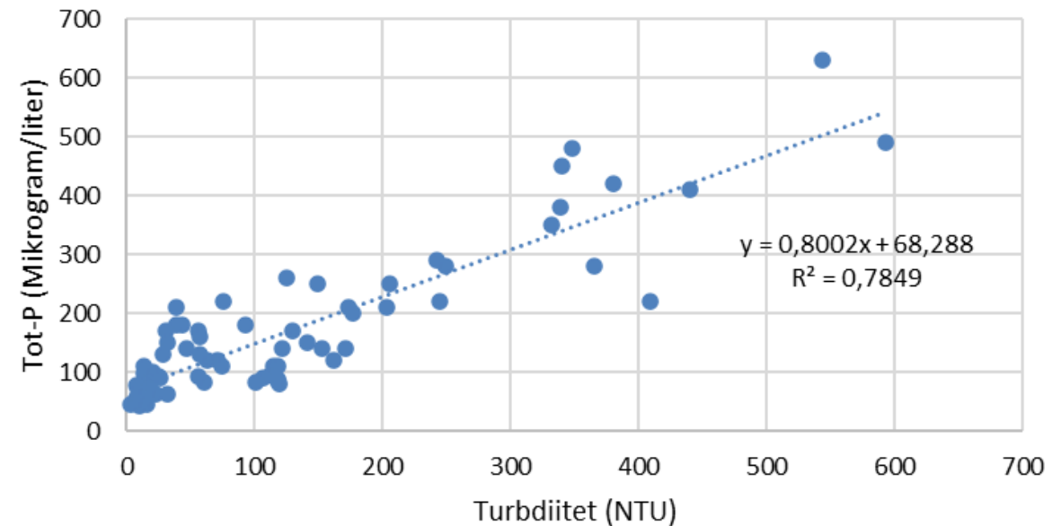
Turbiditet og totalfosfor
