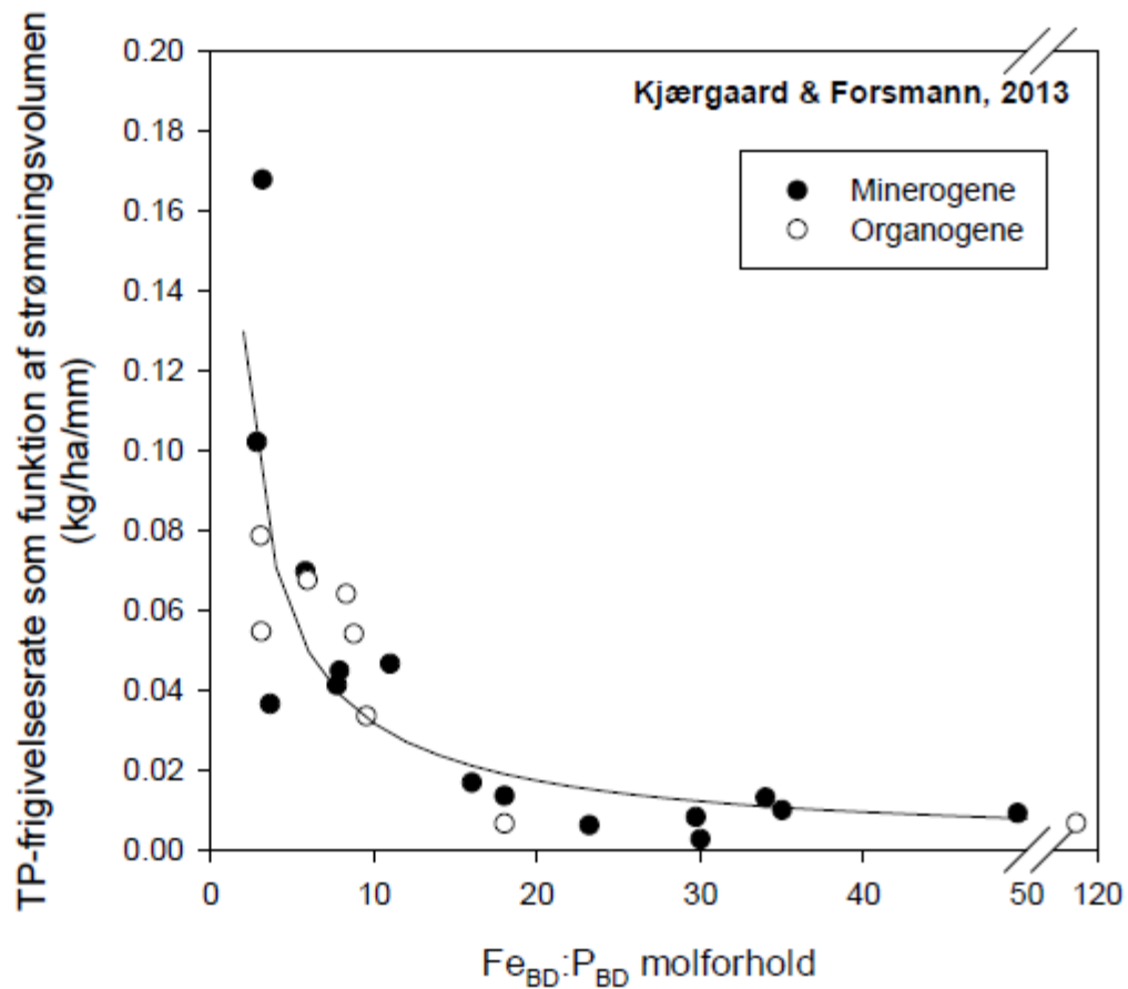
Figur 6.1. TP-frigivelsesrate som funktion af strømningvolumen og jordens Fe_{BD}:P_{BD} -molforhold (kg/ha/mm). Resultater er fra Kjærgaard et al., 2012; Forsmann og Kjærgaard, 2013; Kjærgaard et al., 2013
